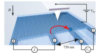
走査ゲート顕微鏡法の原理
