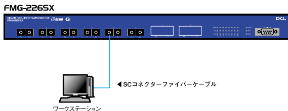
図2-5 コンピュータとの接続
