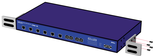
図2-2 ラックマウント用金具の取り付け
