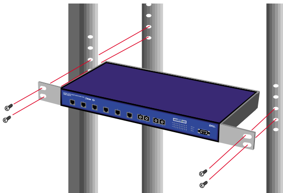
図2-3 ラックへの取り付け
