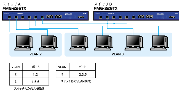
図1-9 「IEEE802.1Qベース」VLAN構成例
