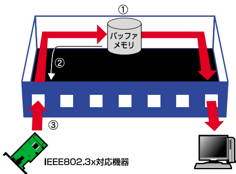
図1-6 フローコントロール
