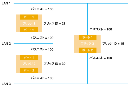
図1-7 STAルールを使用しない場合
