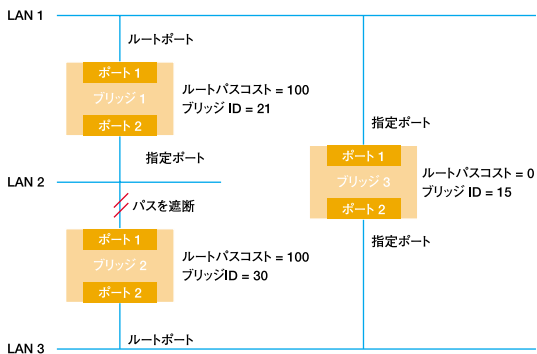
図1-8 STAルールを使用した場合
