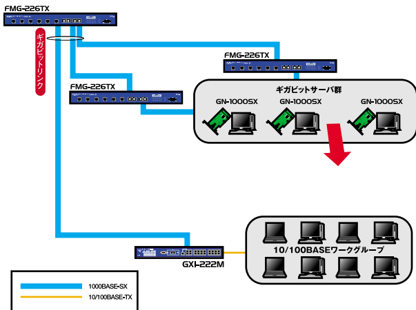
図2-6 ギガビットモジュールを使用したネットワーク
