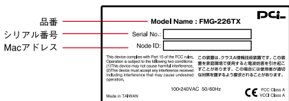
図1-4 裏面ステッカー
