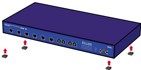
図2-1 ゴム足の取り付け
