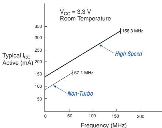
EPM3256A
