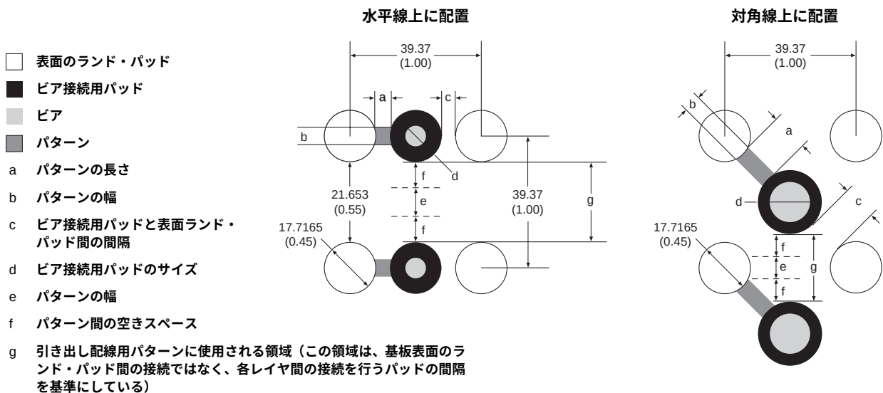
図4 ビア接続用パッドの配置
