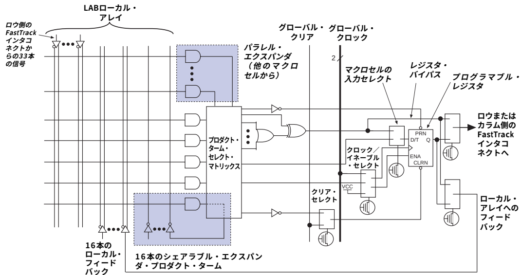
図3 MAX 9000のマクロセルとローカル・アレイ
