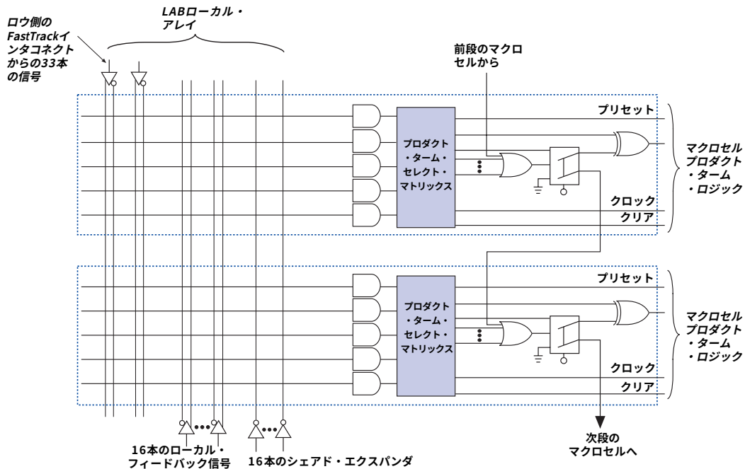
図5 MAX 9000の平行・エクスパンダ
