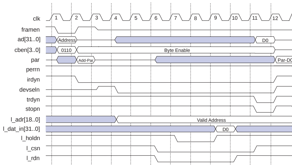
図 7 l_holdnをアサートしたときの外部ターゲット・リード・トランズアクション
