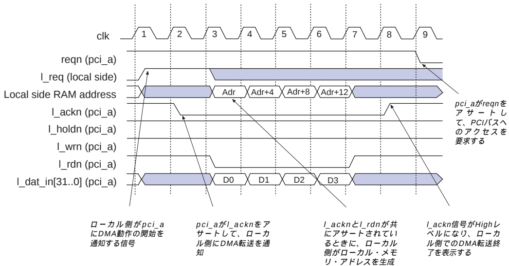
図18 PCIバスDMAライト・トランザクション
